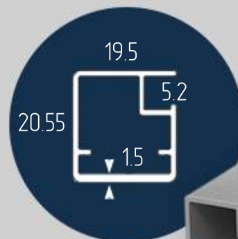
PF-02 ПРОФИЛЬ ФАСАДНЫЙ
